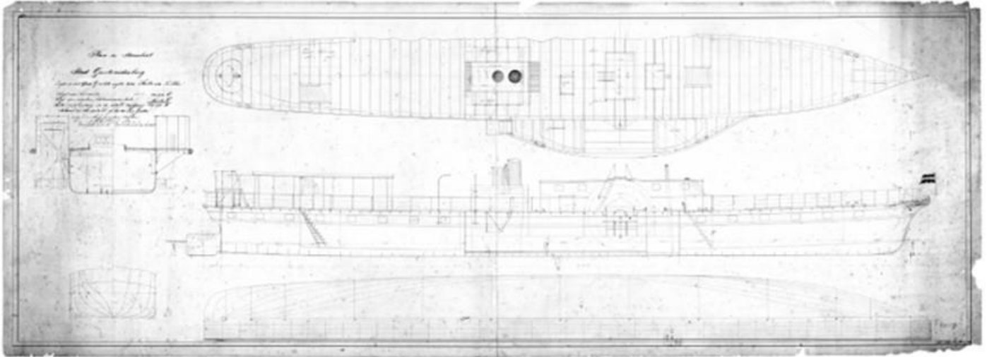
De originele tekening uit 1862 (collectie van het Maritiem museum in Rotterdam)
