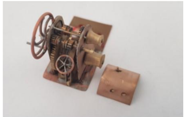
De samengestelde ankerlier zonder kap zodat het binnenwerk goed zichtbaar is.
